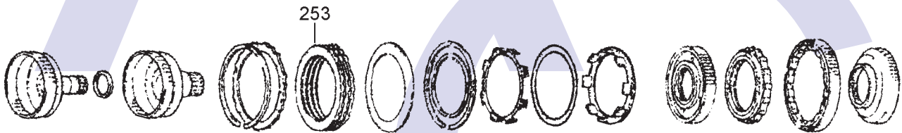
'B3' Brake
